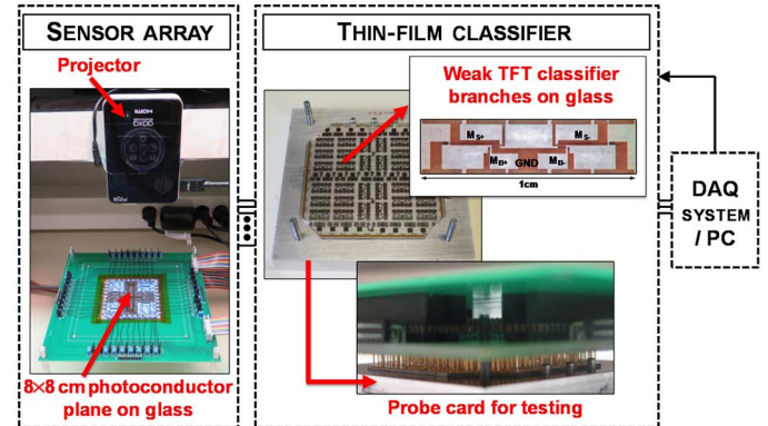
Fig. 15. Thin-film prototype.
